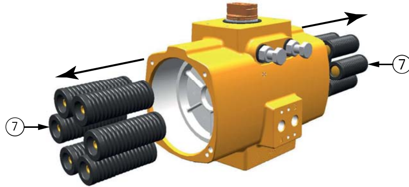
Figure 21 Retrait des cartouches à ressort (tailles 25 à 600)
