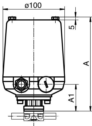
Type d'actionneur B0, B1 avec rehausse métallique
