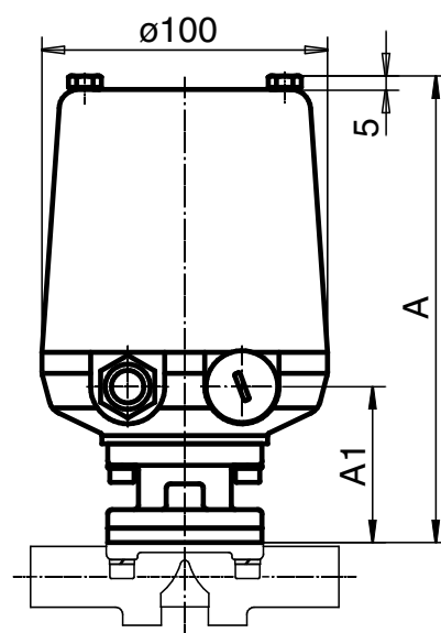
Type d'actionneur B0, B1 avec rehausse métallique
