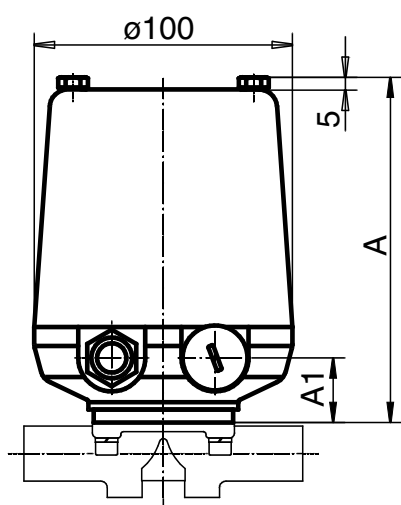
Type d'actionneur A0, A1 Montage direct
