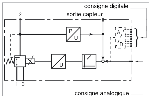
TYPE 614357 - Alimentation interne du capteur de pression
