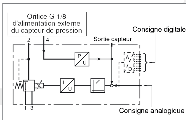
TYPE 614359 - Alimentation externe du capteur de pression
